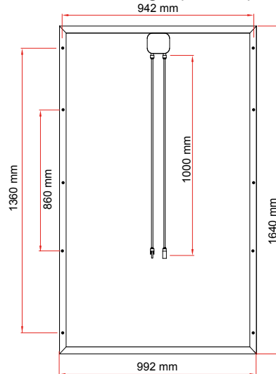
Paneel afmetingen (unit: mm)
