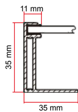
Frame afmetingen (unit: mm)
